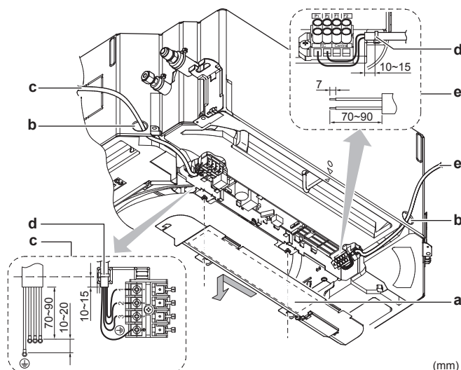
a Huoltokansi (takana kytkentäkaavio) b Kaapelien aukko c Yhteiskytentäkaapelin liittäminen (sisältää maadoituksen) d Nippuside
