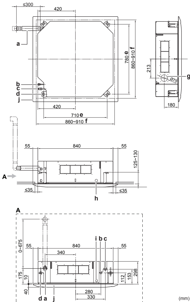
Asennus vakiopaneelin kanssa
