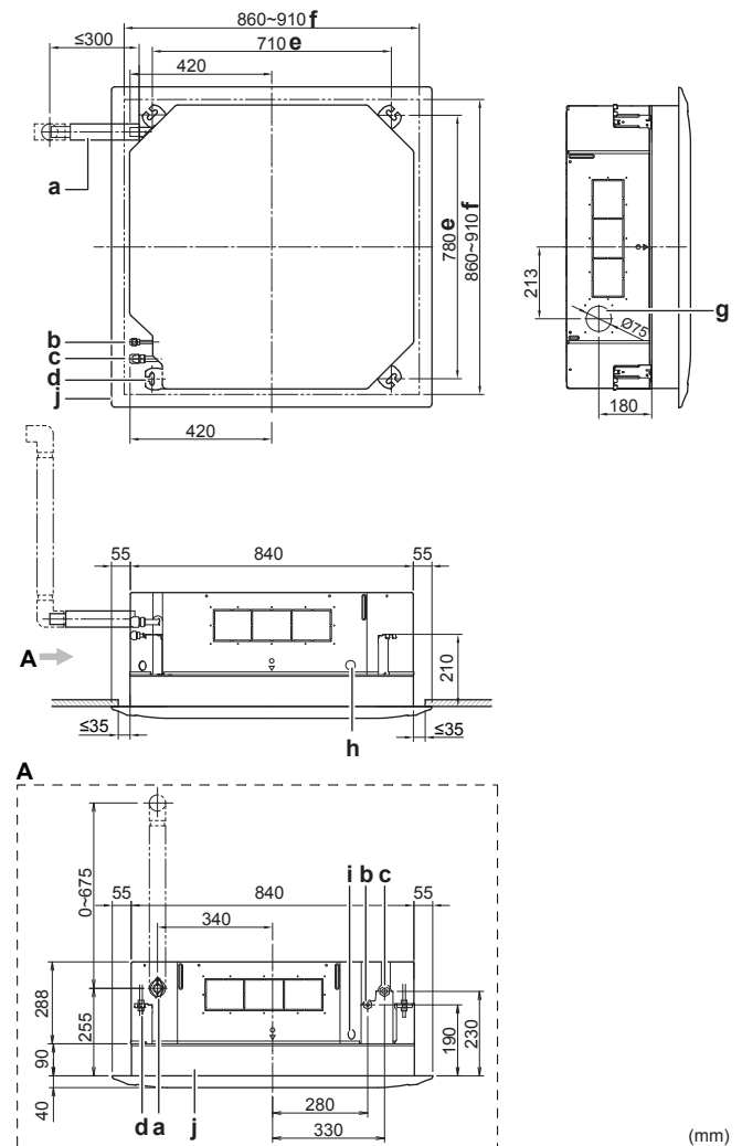
Asennus itse puhdistuvan koristepaneelin kanssa
