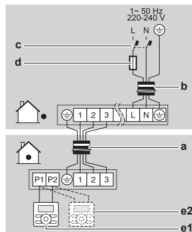
a Yhteiskytentäkaapeli b Virtakaapeli c Maavuotosuojakatkaisin d Sulake e1 Pääkaukosäädin e2 Valinnainen kaukosäädin
